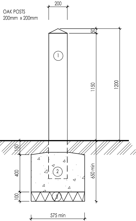
ELEVATION
