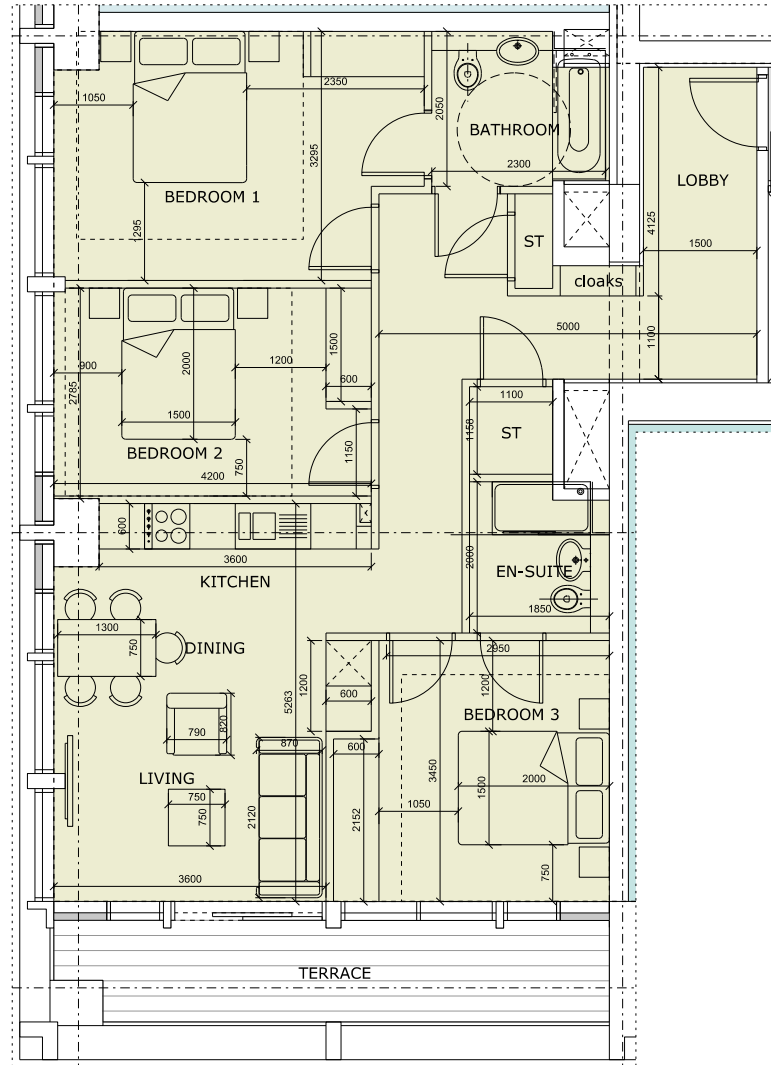
Type E - 3 Bedroom
