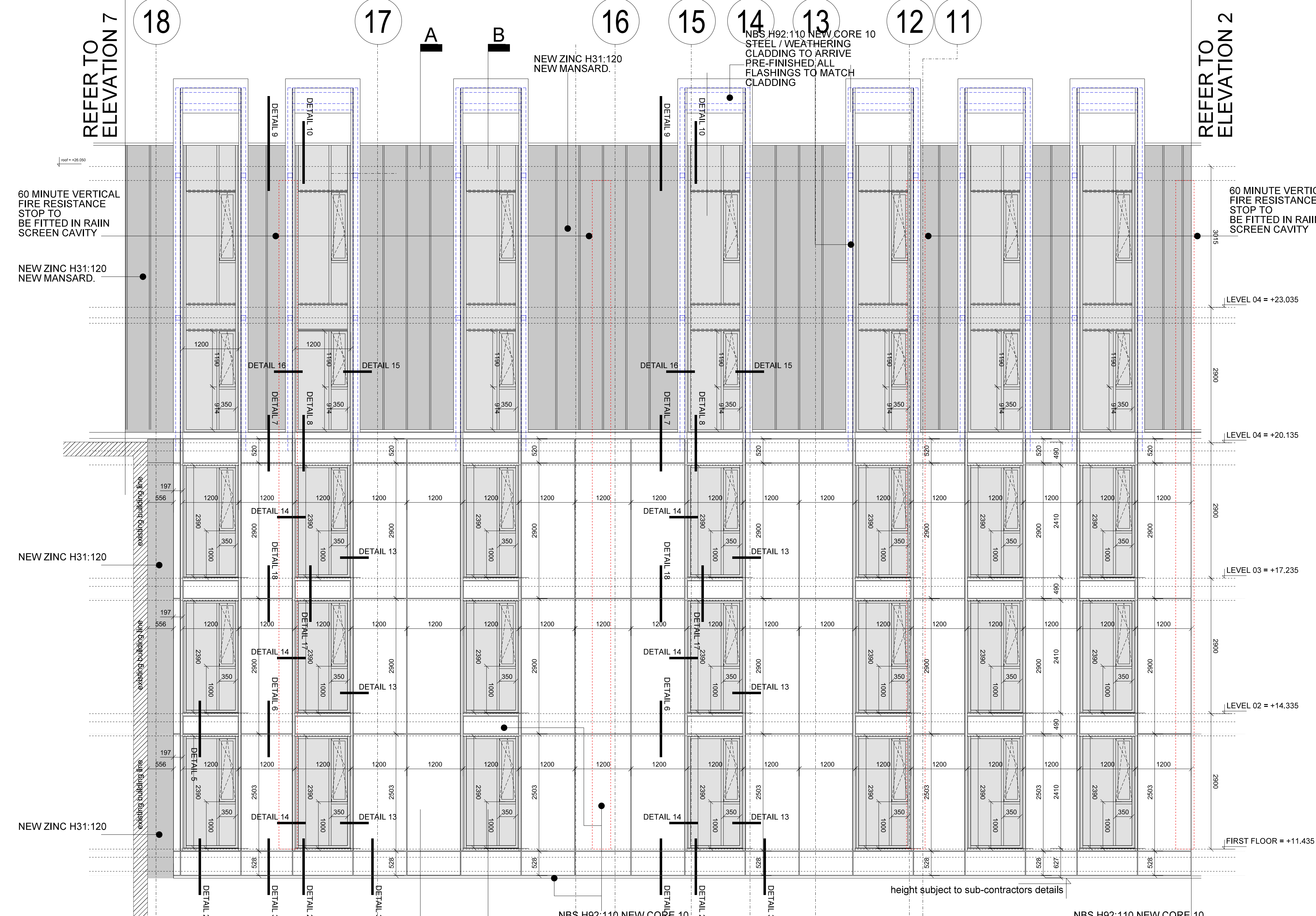
ELEVATION 01
