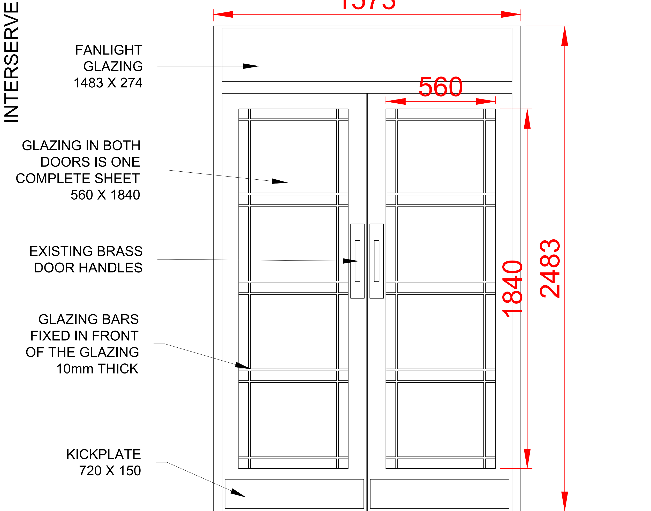
EXISTING 'SUITE A' DOOR 1:10 ELEVATION
