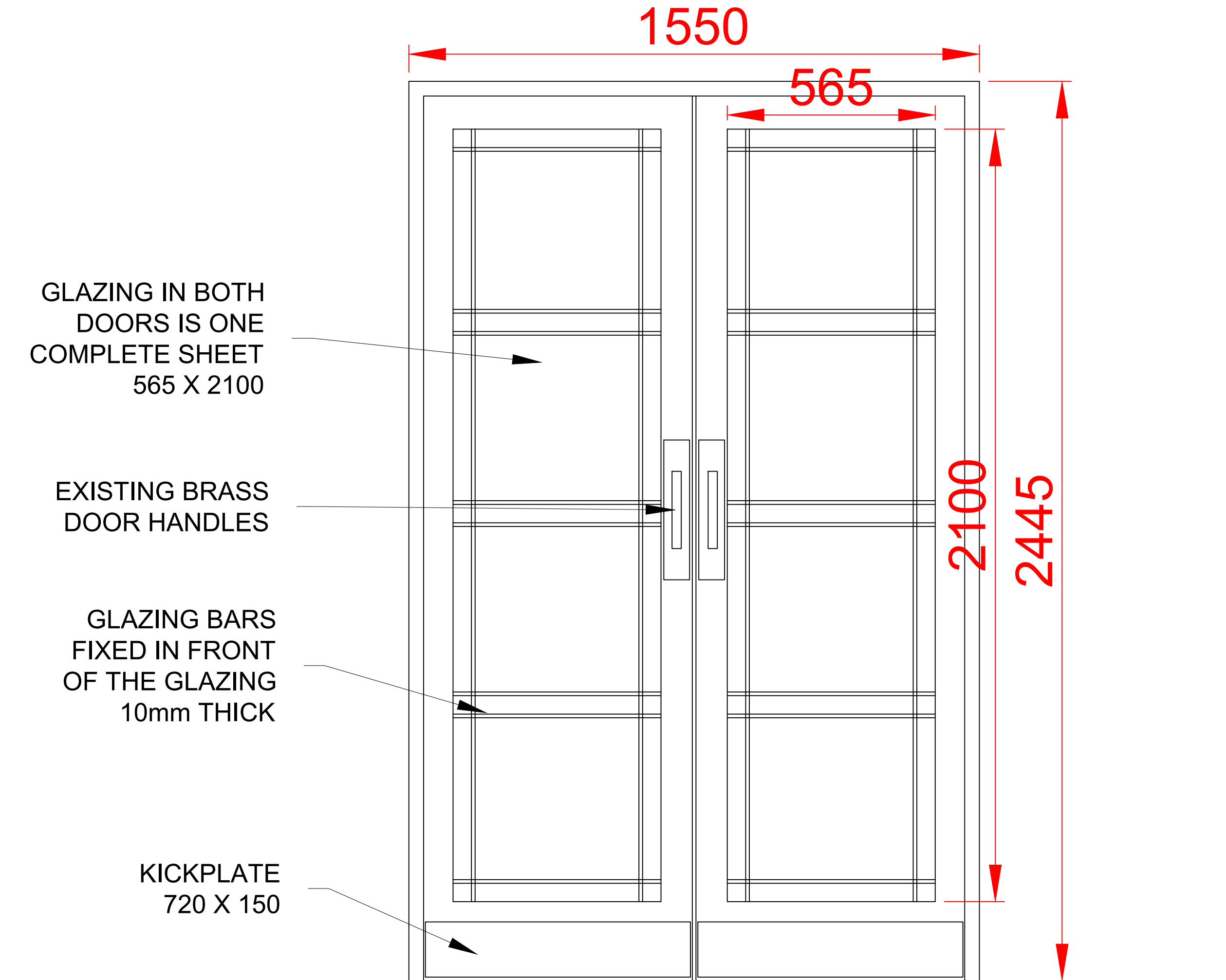
EXISTING 'SUITE B' DOOR 1:10 ELEVATION
