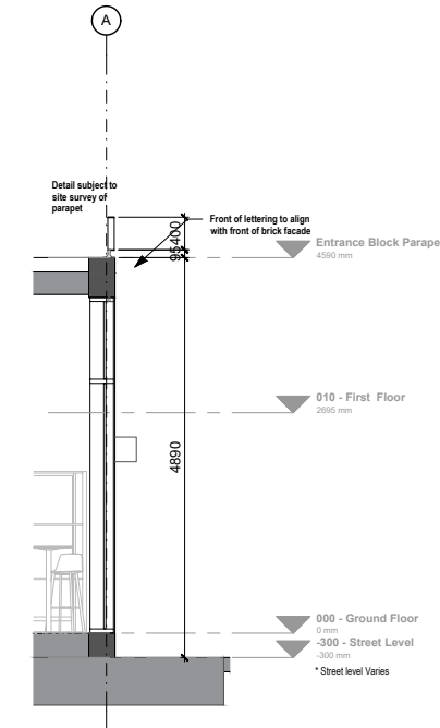
2 Section 1 : 50
