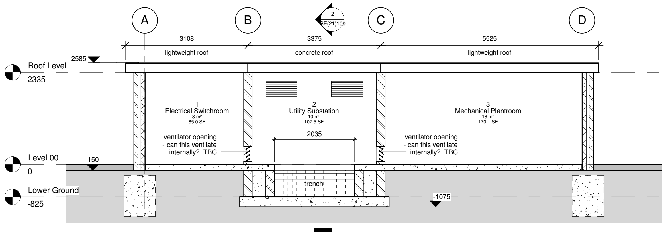
1 Section A-A 1 : 50
