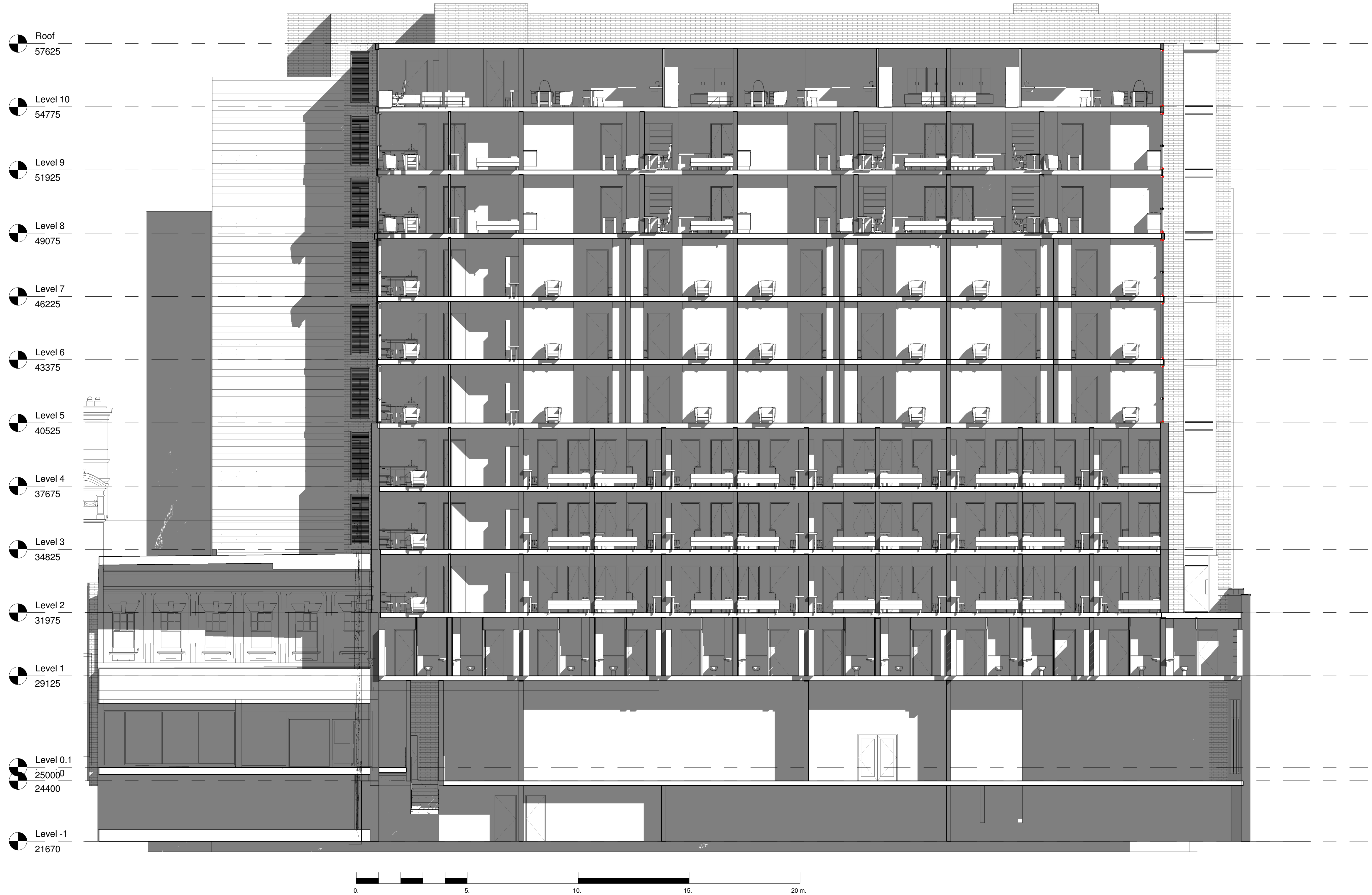
1 03 Section C-C 1 : 100
