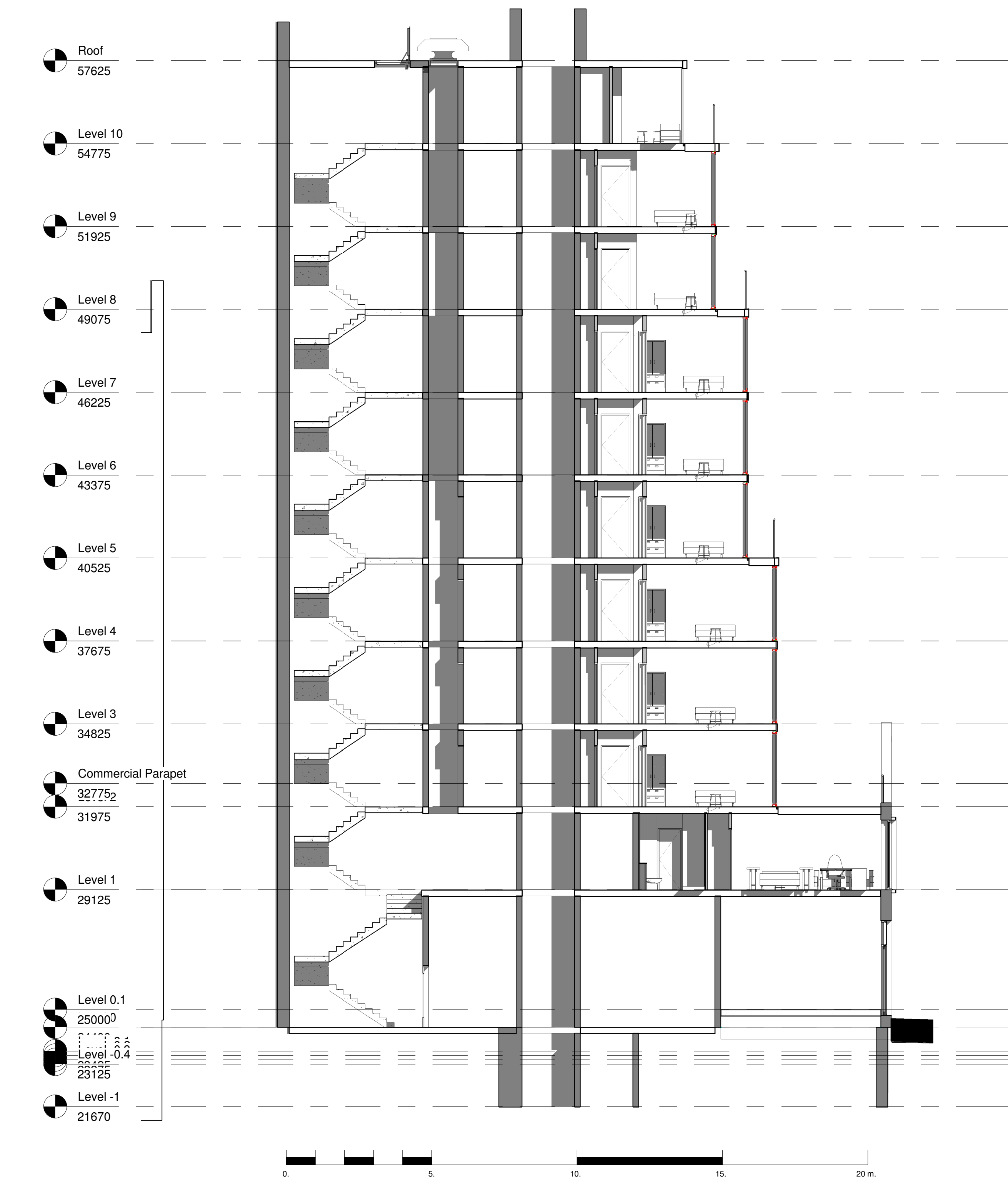
1 01 Section A-A 1 : 100
