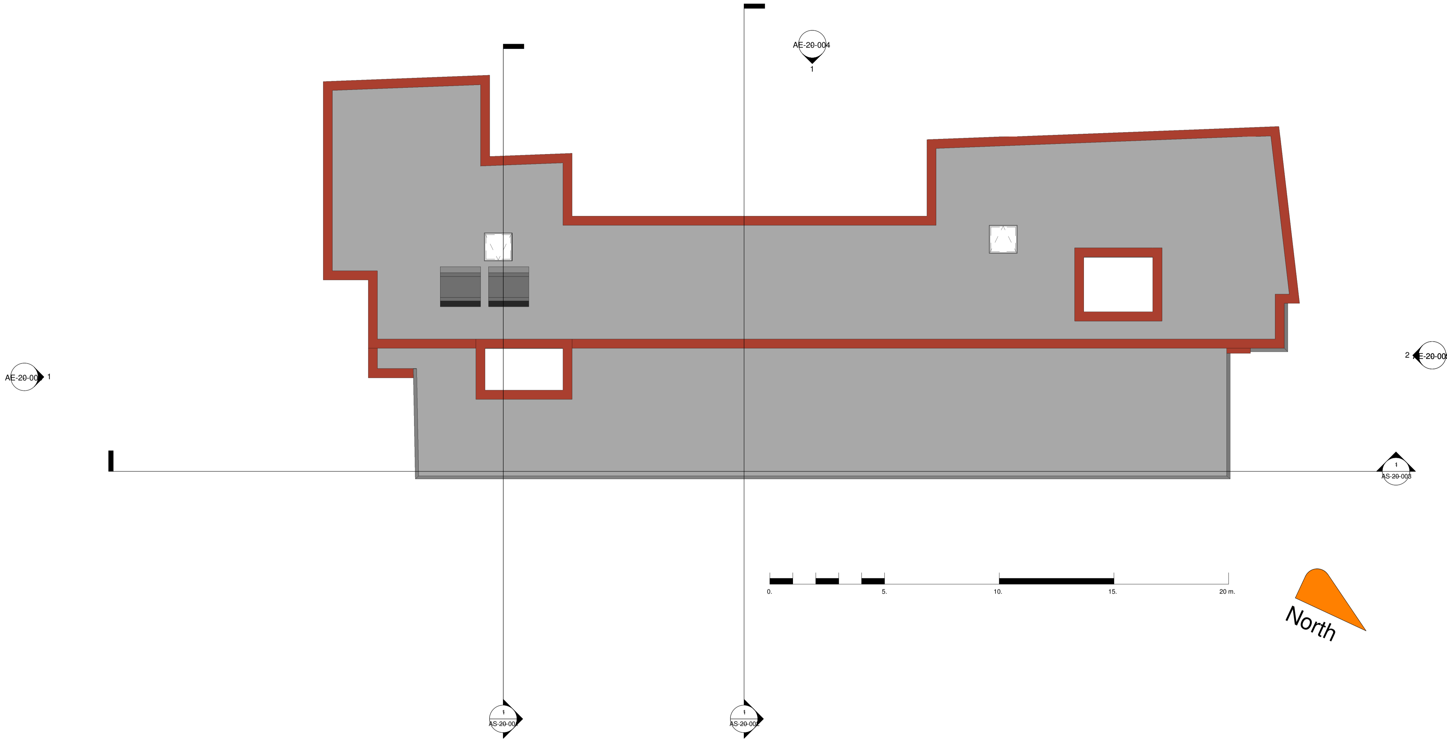
1 Roof Plan 1 : 100
