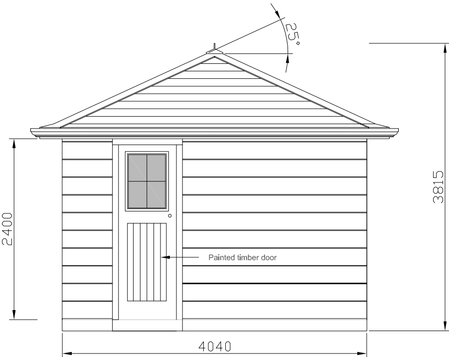
END ELEVATION
